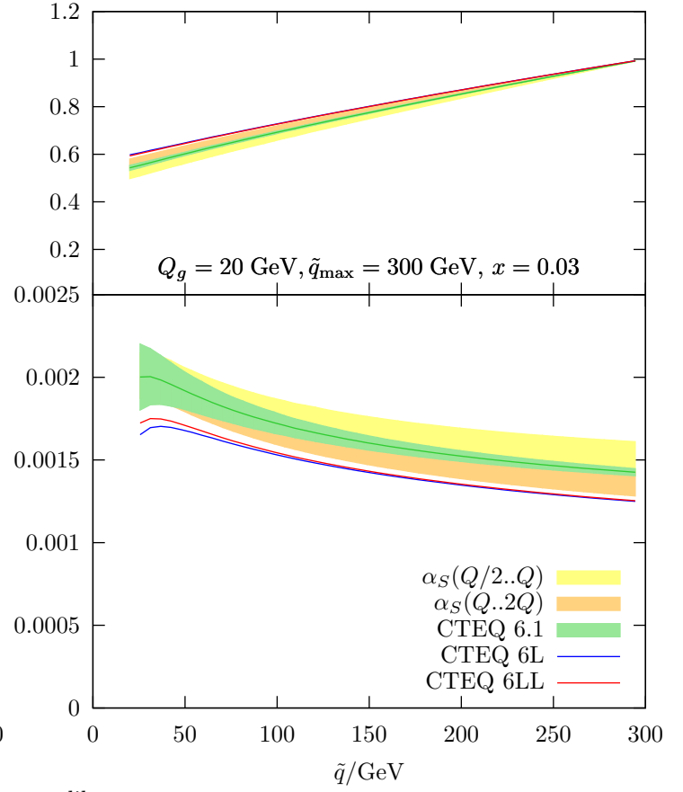
Herwig++ spacelike g \rightarrow gg
