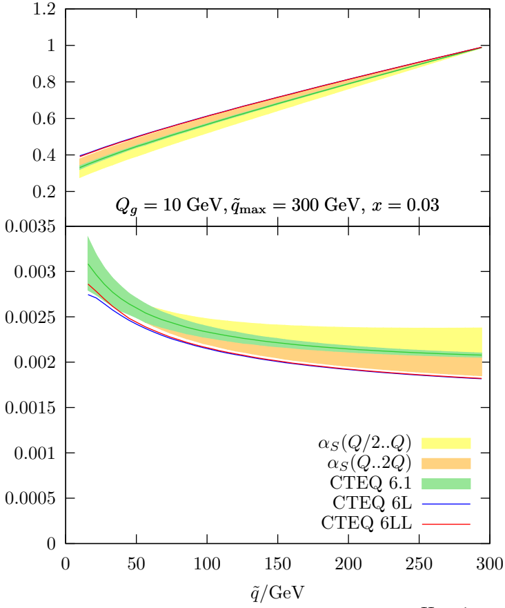
Herwig++ spacelike g \rightarrow gg
