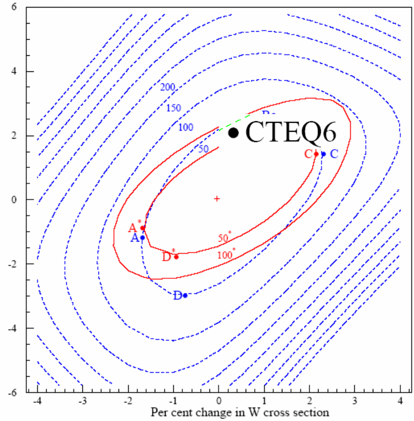
LHC
